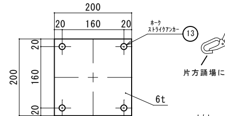
支柱プレート C 矢視
