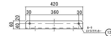
梯子アンカープレート D 矢視
