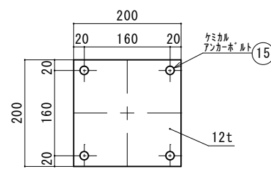
支柱プレート C 矢視
