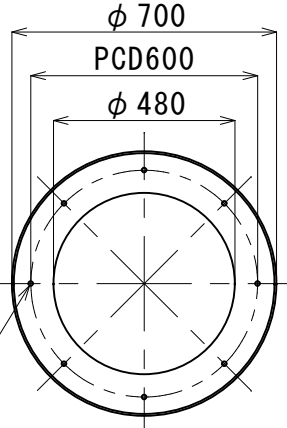
吐出口詳細 S=1/20
