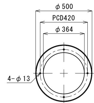
吐出口詳細 S=1/15
