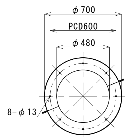
吐出口詳細 S=1/20
