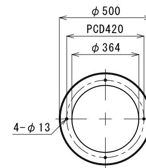
吐出口詳細 S=1/15
